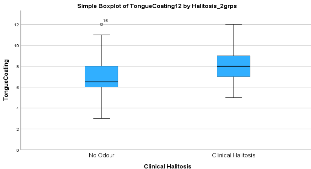
RAJAH 2. Rajah kotak membandingkan tahap lapisan permukaan lidah antara peserta dengan dan tanpa halitosis klinikal
